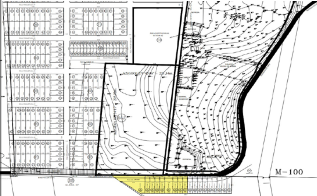
PLANTA DA QUADRA Nº 102 - SETOR 15 ESCALA: 1:1.000
